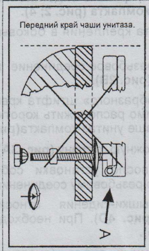
Рис. 3. Неправильная установка. Незастыгший вид.
