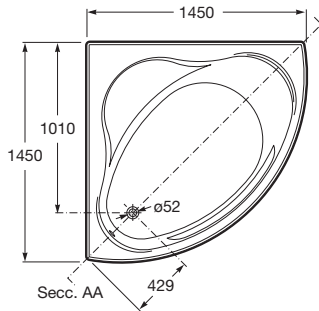
Secc. AA
