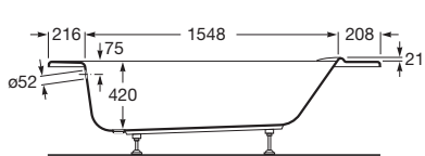
Secc. AA
