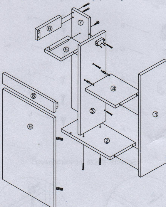
Rys.3. Szafka w wersji prawej
