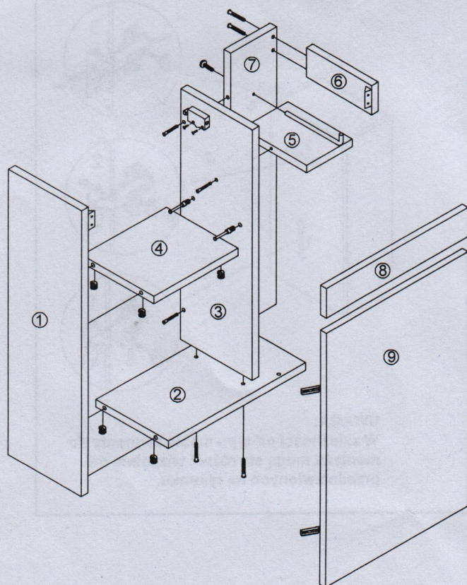
Rys.1. Szafka w wersji lewej
