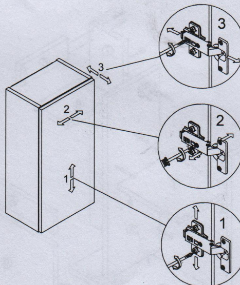
Rys.4. Regulacja ustawień drzwiczek.
