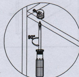
Schemat złącza mimośrodowego
