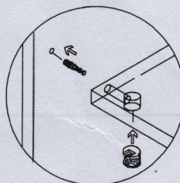
Schemat złącza mimośrodowego
