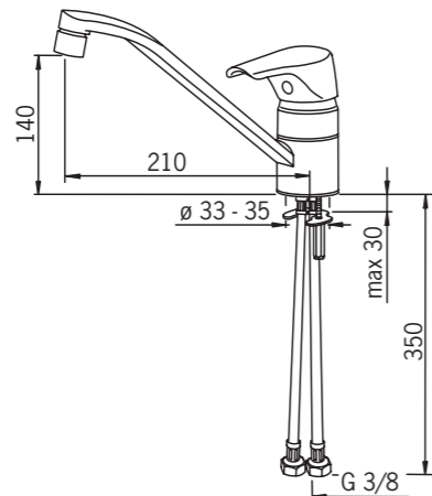
1930F Oras Saga для кухни
