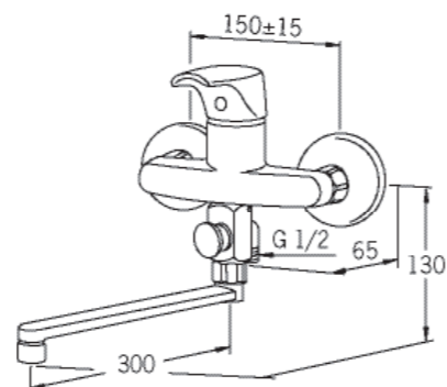
1942Y Oras Saga для ванны и душа
