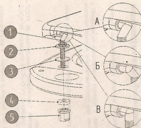
Рис.1 - Установка арматуры крепления
