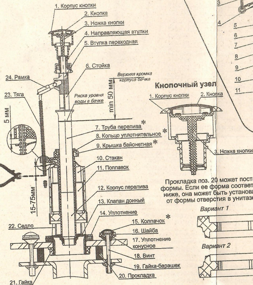
Рис. 2 - Клапан выпуска
