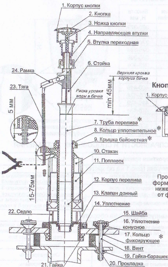
Рис. 2 - Клапан выпуска
